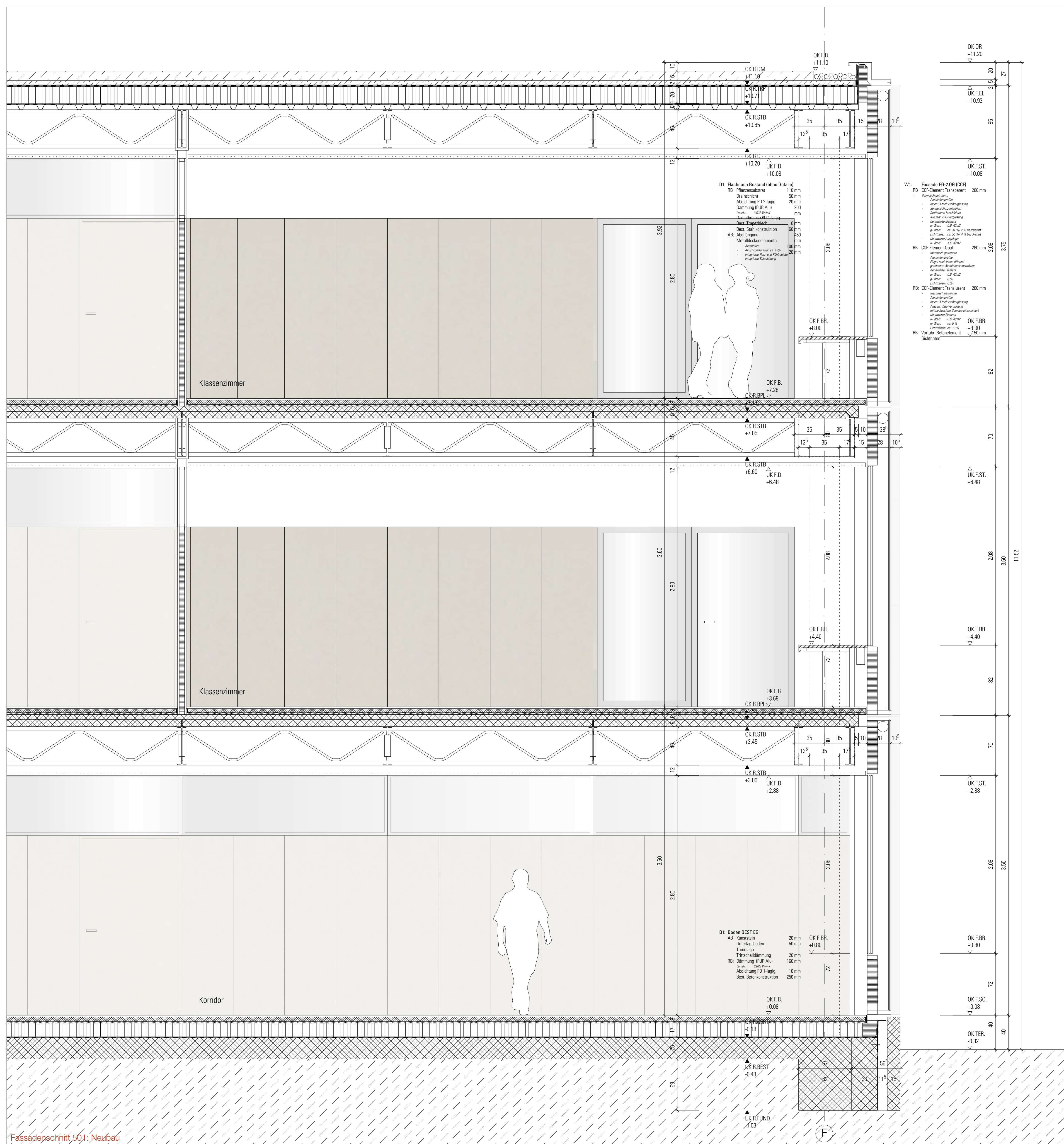
Fassadenschnitt 501: Neubau
